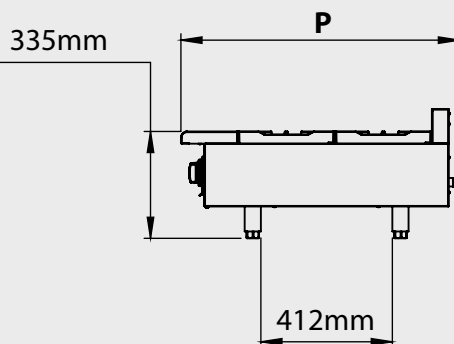
VISTA LATERAL
